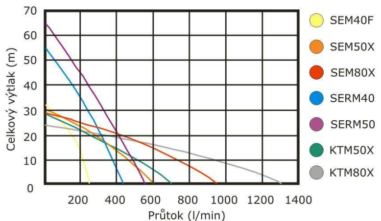
Závislost výtlaku na průtoku
